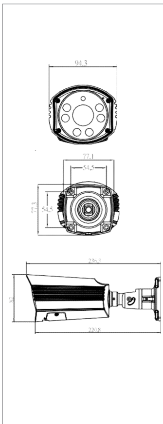
製品寸法 (mm)
